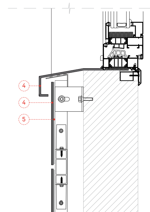
Appuis de fenêtre
