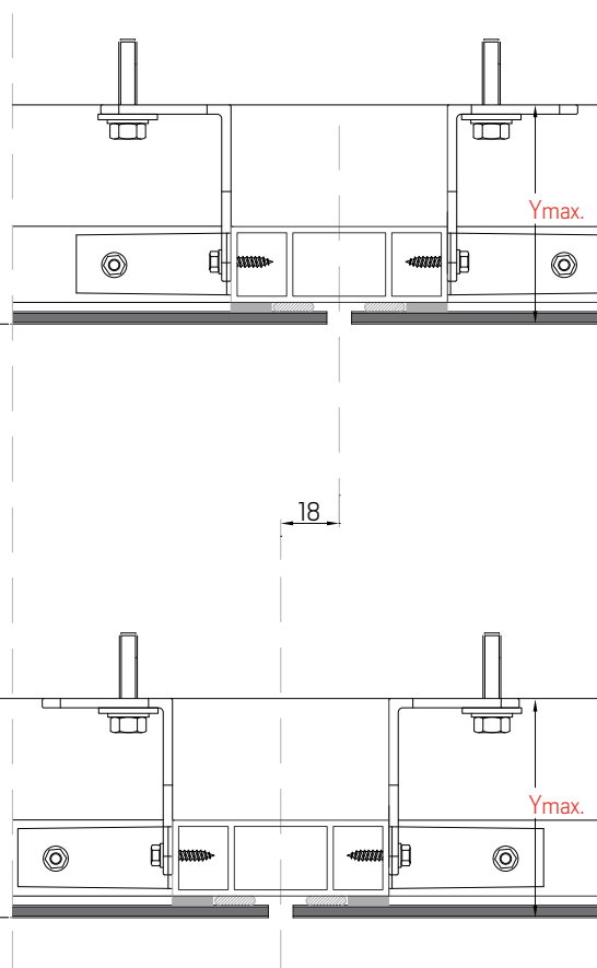
AILES ANCRAGE ANGULAIRE EN AXE Y
