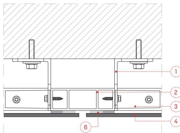
SECTION HORIZONTALE
