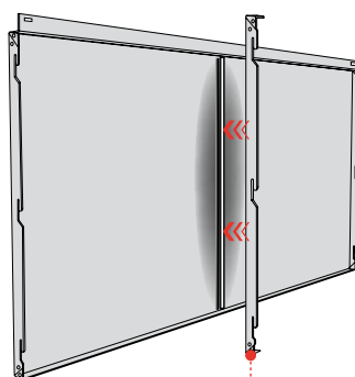
5 COLLER LE RAIDISSEUR
