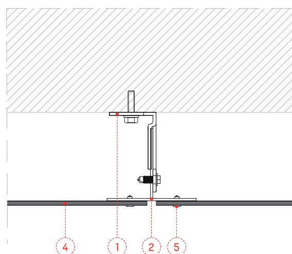
SECTION HORIZONTALE
