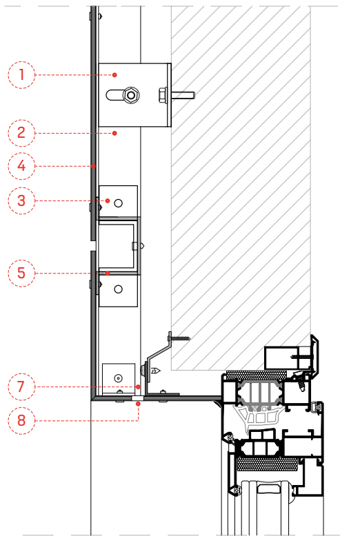
Détail de linteau
