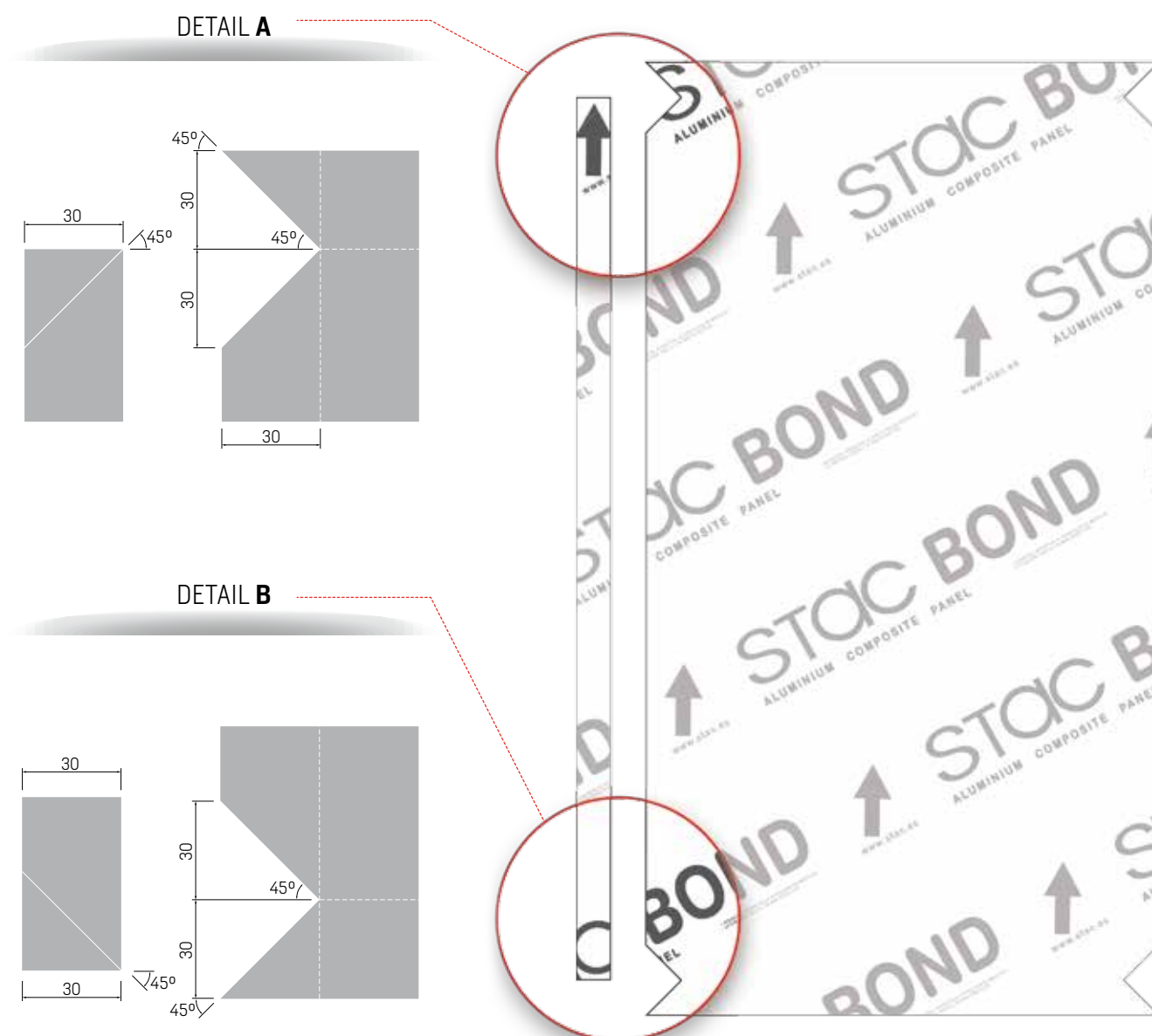
Détail de coupe de panneau
