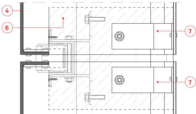
TRAITEMENT DE L'ACCROTÈRE SECTION HORIZONTALE
