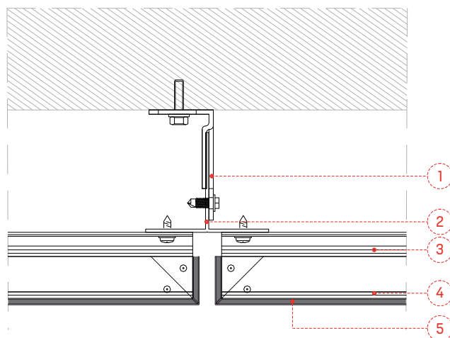
SECTION HORIZONTALE
