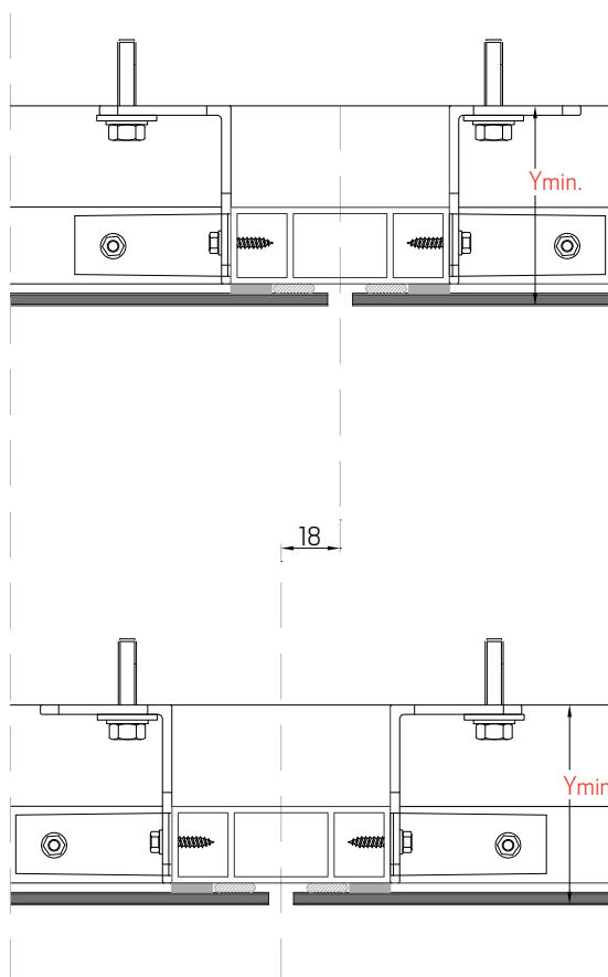
BASE ANCRAGE ANGULAIRE EN AXE X
