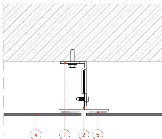
SECTION HORIZONTALE
