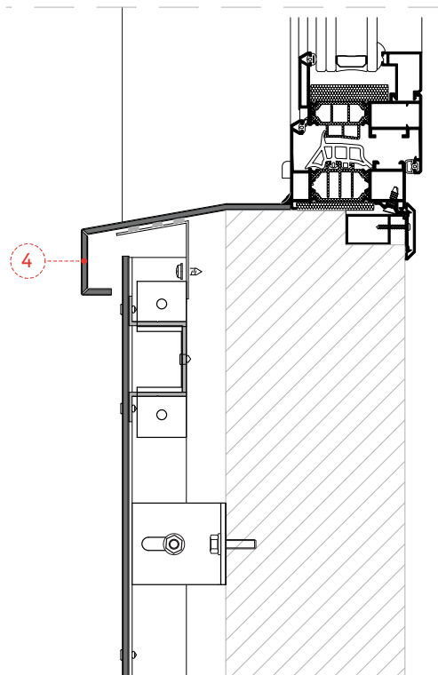
Appuis de fenêtre
