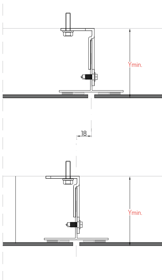
BASE SÉPARATEUR L EN AXE X
