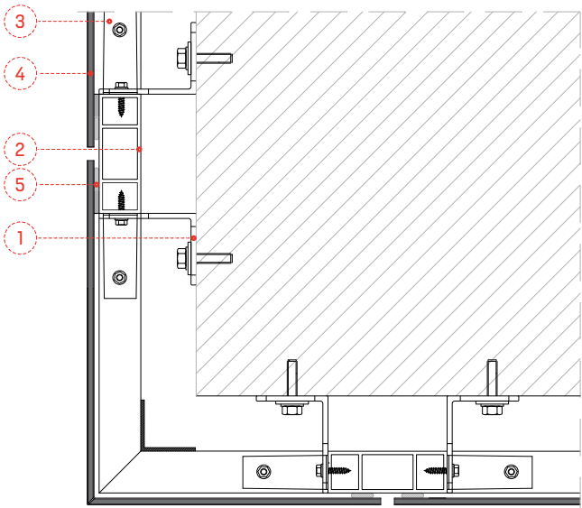
TERMINAISON D'ANGLE SECTION HORIZONTALE
