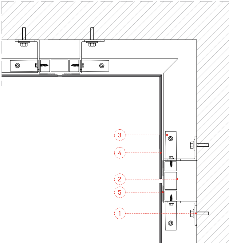
TERMINAISON D'ANGLE SECTION HORIZONTALE
