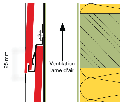
RECouvrement DES PANNEAUX SCALEO
