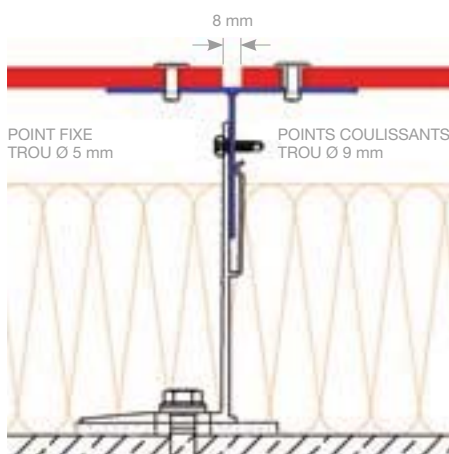
COUPE SUR JOINT VERTICAL
