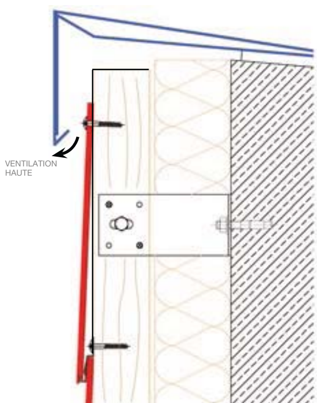
DÉTAIL COUVERTINE
