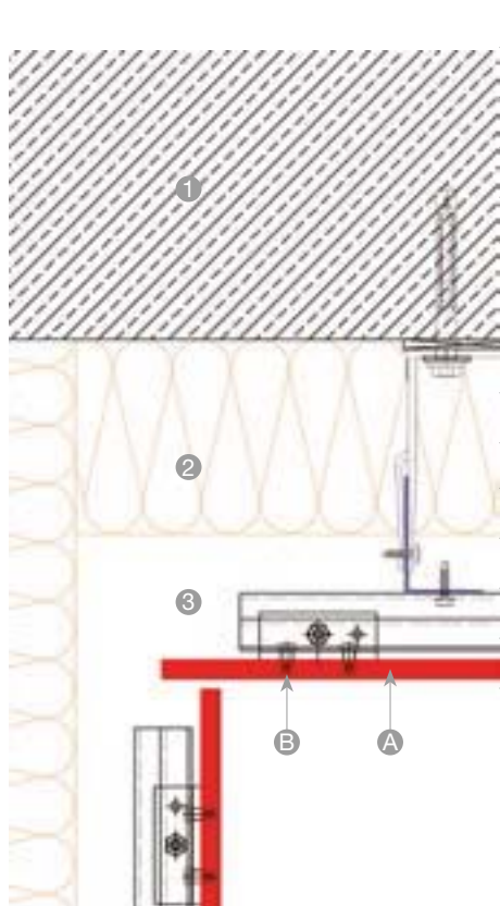
ANGLE RENTRANT
