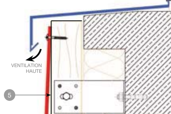
DÉTAIL APPUI DE FENÊTRE
