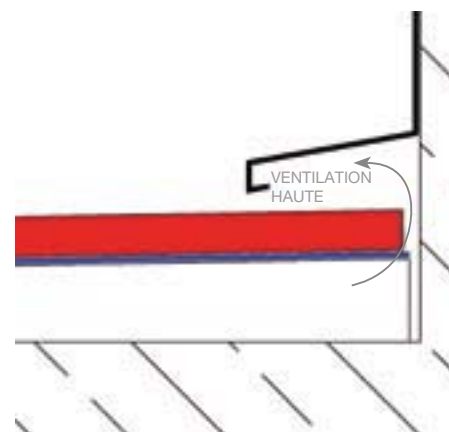
COUPE VERTICALE DU PRINCIPE DE LA JONCTION À LA FAÇADE
