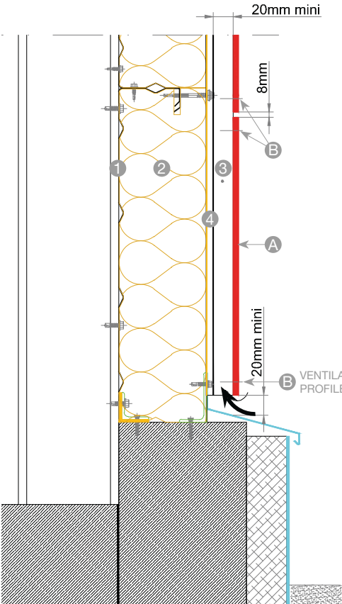
DÉTAILS POINT BAS
