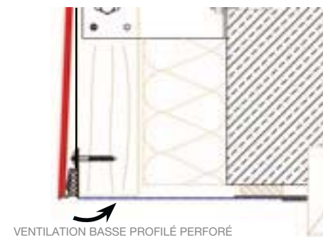
DÉTAIL LINTEAU
