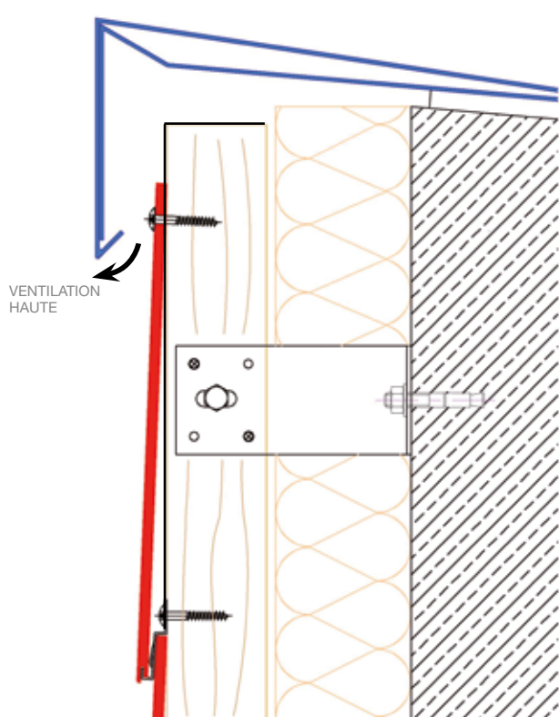
DÉTAIL COUVERTINE
