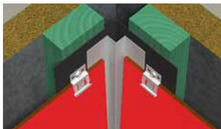
PROFIL D'ANGLE RENTRANT
