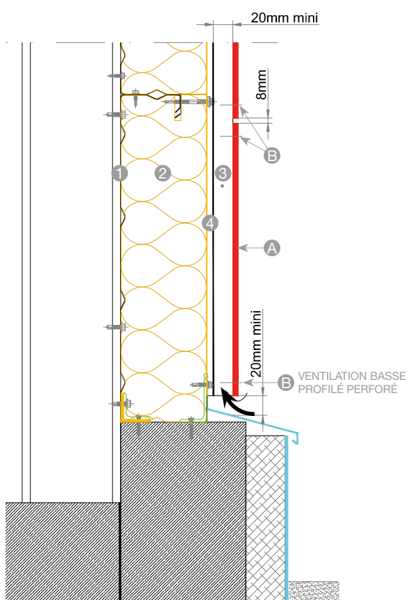
DÉTAILS POINT BAS
