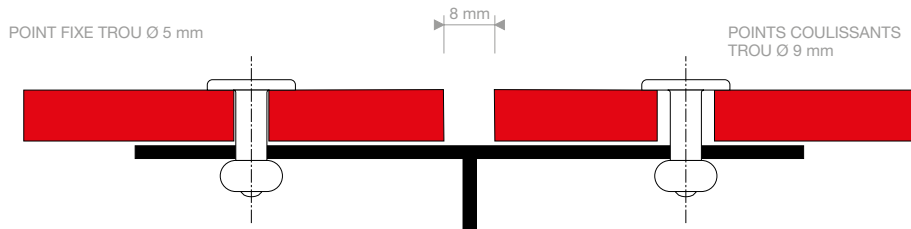
EXEMPLE DE JOINT VERTICAL
