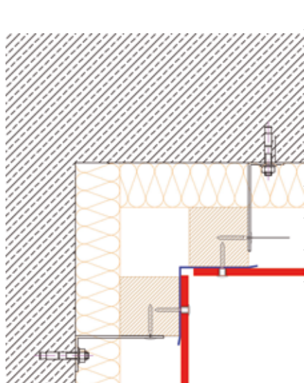
ANGLE RENTRANT
