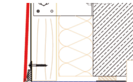
DÉTAIL LINTEAU
