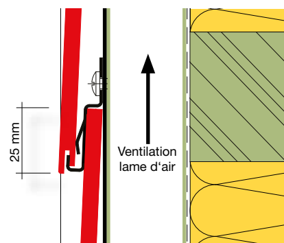
RECOUVREMENT DES PANNEAUX
