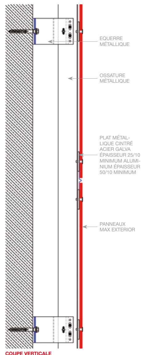
COUPE VERTICALE
